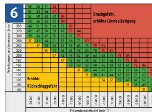
Drehzahlen aus dem grünen Bereich des Diagramms wählen.
