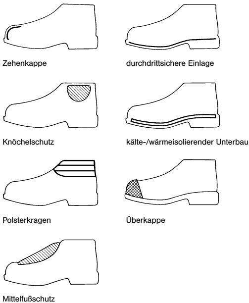
Bild 2: Beispiele für sicherheitstechnische Ausrüstungen beim Fußschutz
