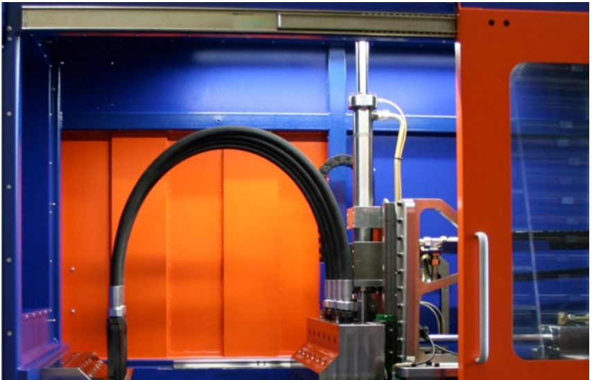
Abb. 3 Impuls-Prüfstand beim Schlauchleitungshersteller
