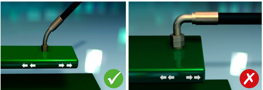
Abb. 16 Verlegung bei Schwingungen
