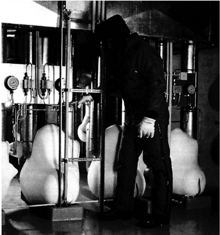
Abb. 10: Ausführungsbeispiel für Kälteschutzkleidung
