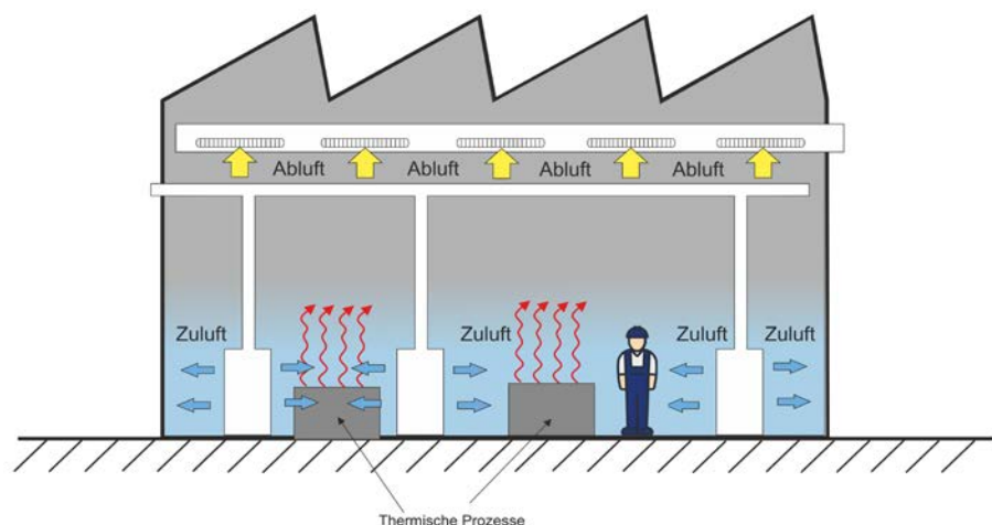
Abb. 5 Prinzip Schichtströmung
