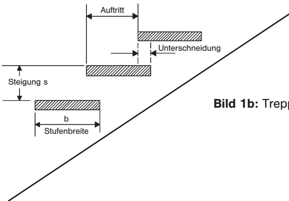
Bild 1: Maßbegriffe einer Treppe
