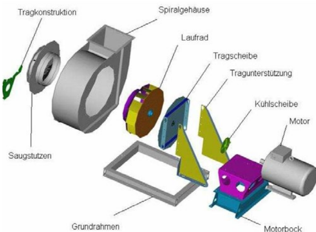
Abb. 3.4.5 Einzelteile eines direkt angetriebenen Radialventilators
