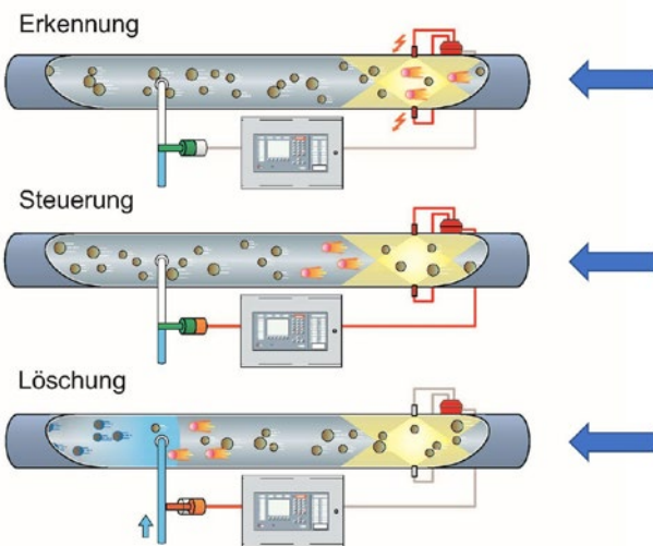
Abb. 3.9.2 Bestandteile und Wirkungsweise einer Funken-detections- und -löschanlage
