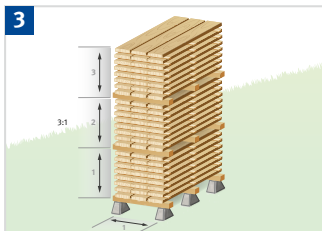
Einzel stehende Pakete unbesäumter Ware zum Trocknen im Freien. Die Lagen sind nicht voll ausgefüllt, deshalb darf das Verhältnis Höhe zu Breite max. 3:1 sein.
