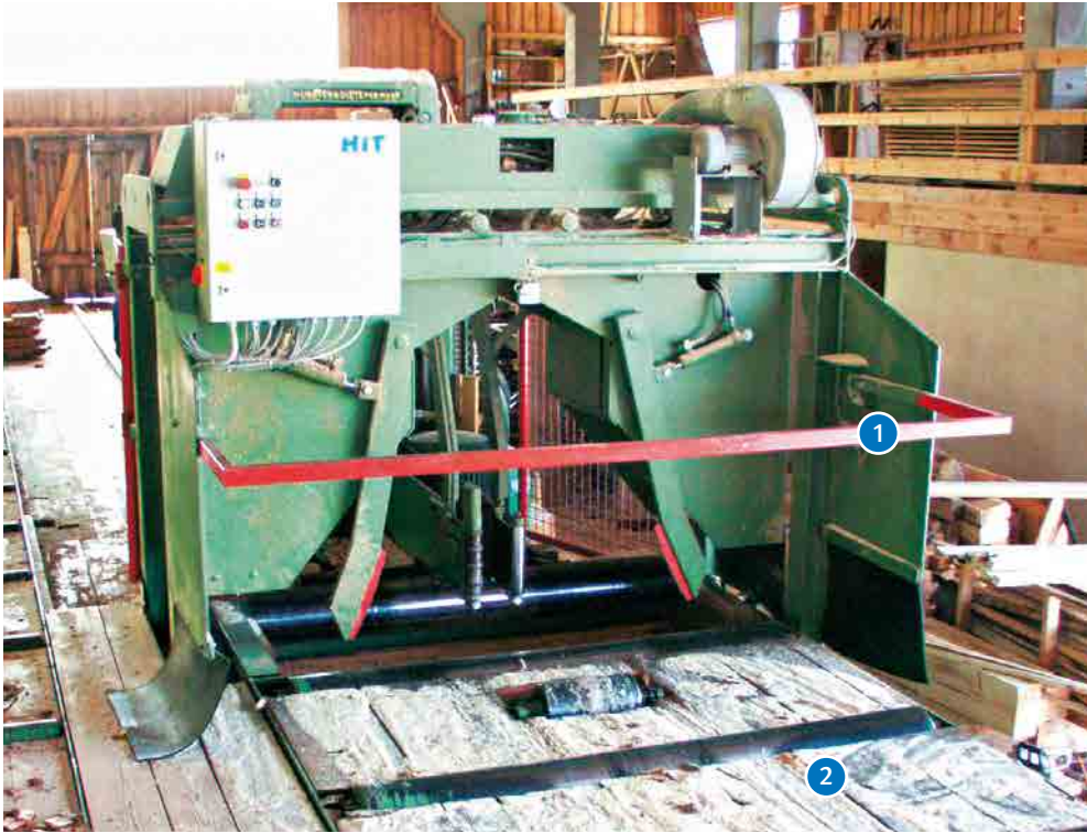
Abb. 9 Seitenwarenkappanlage – Ausschubbereich
