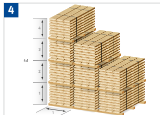
Im Freien nebeneinandergesetzte Schnittholz-Kastenstapel-Pakete mit voll ausgefüllten Lagen, bei besäumter Ware, Verhältnis Höhe zu Breite max. 4:1, max. 5 m hoch.
